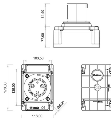
ГАБАРИТНЫЙ ЧЕРТЁЖ
