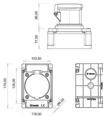
ГАБАРИТНЫЙ ЧЕРТЁЖ
