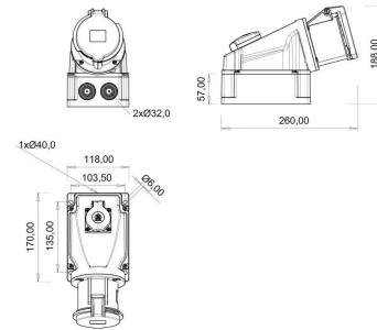
ГАБАРИТНЫЙ ЧЕРТЁЖ
