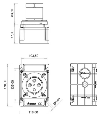
ГАБАРИТНЫЙ ЧЕРТЁЖ
