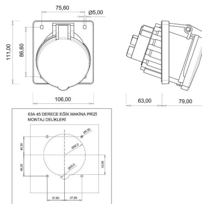
ГАБАРИТНЫЙ ЧЕРТЁЖ
