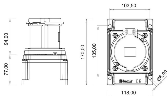
ГАБАРИТНЫЙ ЧЕРТЁЖ
