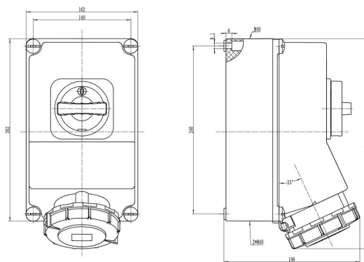
ГАБАРИТНЫЙ ЧЕРТЁЖ
