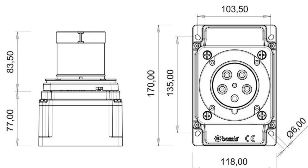
ГАБАРИТНЫЙ ЧЕРТЁЖ
