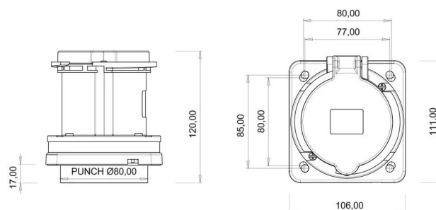
ГАБАРИТНЫЙ ЧЕРТЁЖ
