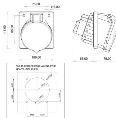
ГАБАРИТНЫЙ ЧЕРТЁЖ
