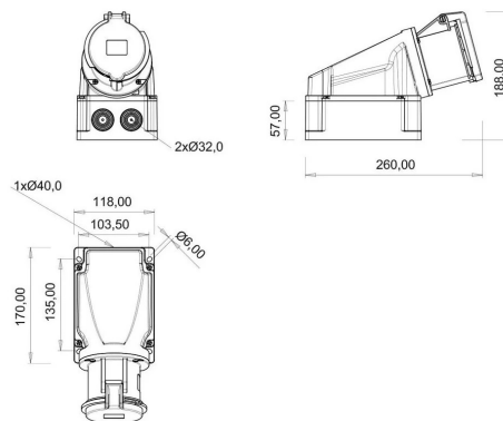
ГАБАРИТНЫЙ ЧЕРТЁЖ
