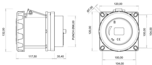
ГАБАРИТНЫЙ ЧЕРТЁЖ
