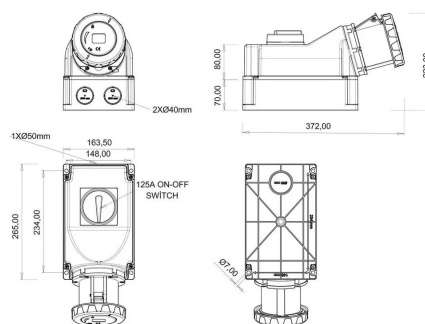
ГАБАРИТНЫЙ ЧЕРТЁЖ
