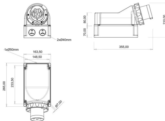
ГАБАРИТНЫЙ ЧЕРТЁЖ
