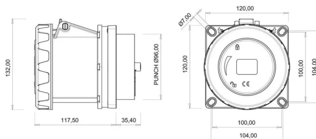
ГАБАРИТНЫЙ ЧЕРТЁЖ
