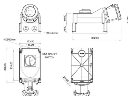
ГАБАРИТНЫЙ ЧЕРТЁЖ
