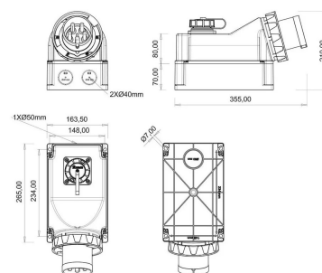
ГАБАРИТНЫЙ ЧЕРТЁЖ
