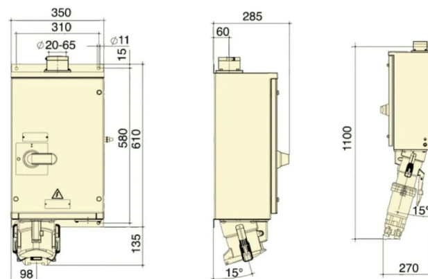
ГАБАРИТНЫЙ ЧЕРТЁЖ
