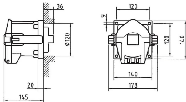
ГАБАРИТНЫЙ ЧЕРТЁЖ
