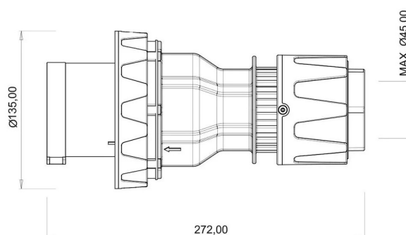
ГАБАРИТНЫЙ ЧЕРТЁЖ
