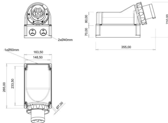
ГАБАРИТНЫЙ ЧЕРТЁЖ
