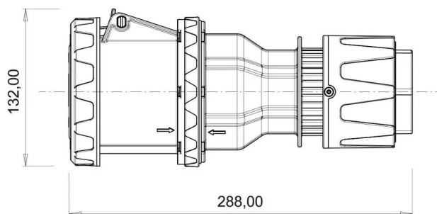
ГАБАРИТНЫЙ ЧЕРТЁЖ
