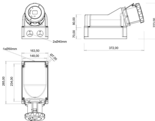
ГАБАРИТНЫЙ ЧЕРТЁЖ
