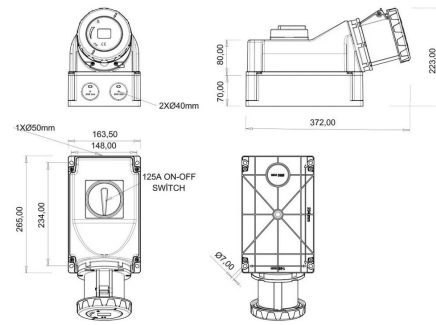
ГАБАРИТНЫЙ ЧЕРТЁЖ
