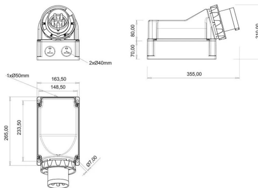
ГАБАРИТНЫЙ ЧЕРТЁЖ
