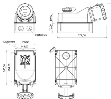
ГАБАРИТНЫЙ ЧЕРТЁЖ
