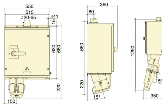
ГАБАРИТНЫЙ ЧЕРТЁЖ
