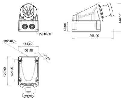
ГАБАРИТНЫЙ ЧЕРТЁЖ
