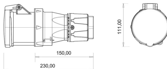
ГАБАРИТНЫЙ ЧЕРТЁЖ
