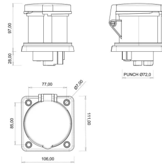
ГАБАРИТНЫЙ ЧЕРТЁЖ
