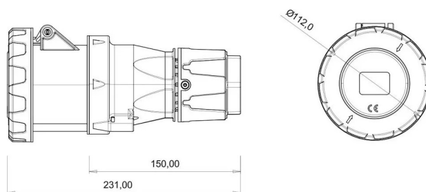
ГАБАРИТНЫЙ ЧЕРТЁЖ
