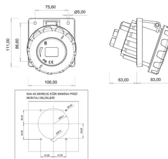
ГАБАРИТНЫЙ ЧЕРТЁЖ
