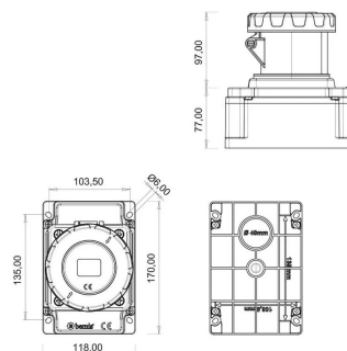
ГАБАРИТНЫЙ ЧЕРТЁЖ
