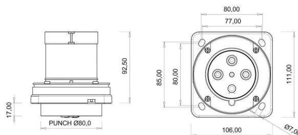
ГАБАРИТНЫЙ ЧЕРТЁЖ
