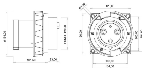
ГАБАРИТНЫЙ ЧЕРТЁЖ
