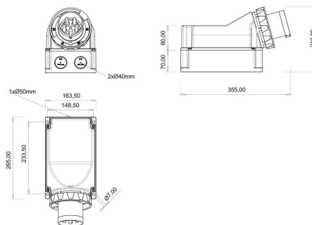
ГАБАРИТНЫЙ ЧЕРТЁЖ
