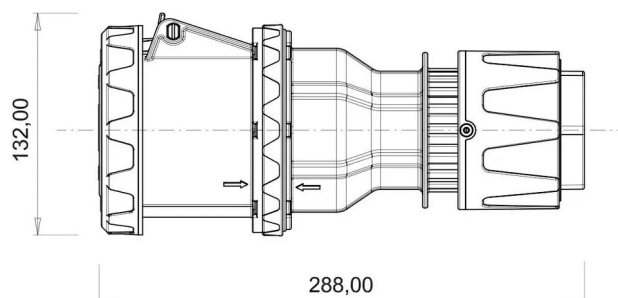
ГАБАРИТНЫЙ ЧЕРТЁЖ
