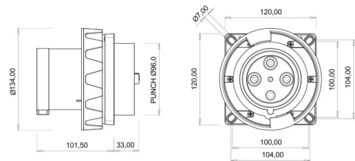
ГАБАРИТНЫЙ ЧЕРТЁЖ
