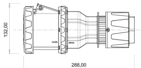
ГАБАРИТНЫЙ ЧЕРТЁЖ
