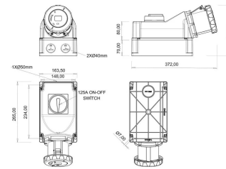
ГАБАРИТНЫЙ ЧЕРТЁЖ
