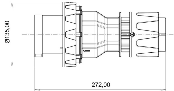
ГАБАРИТНЫЙ ЧЕРТЁЖ
