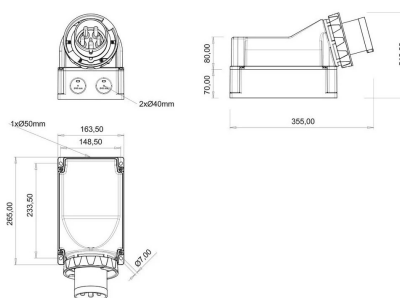
ГАБАРИТНЫЙ ЧЕРТЁЖ
