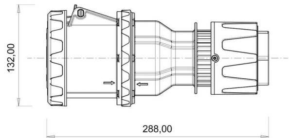
ГАБАРИТНЫЙ ЧЕРТЁЖ
