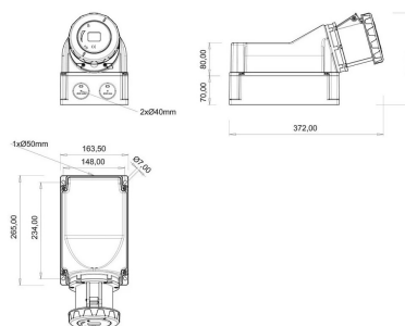
ГАБАРИТНЫЙ ЧЕРТЁЖ
