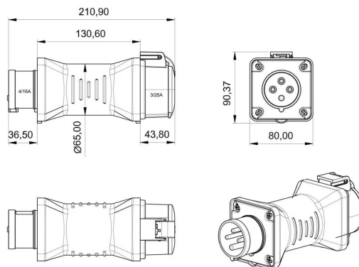
ГАБАРИТНЫЙ ЧЕРТЁЖ
