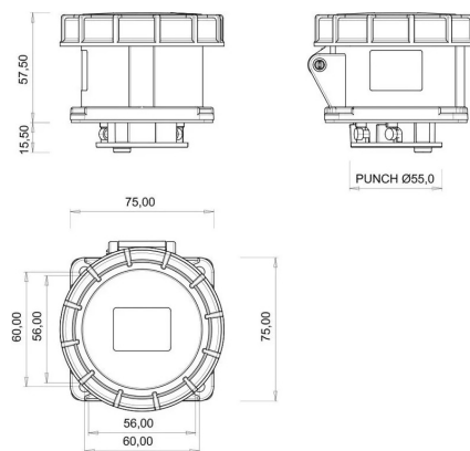
ГАБАРИТНЫЙ ЧЕРТЁЖ
