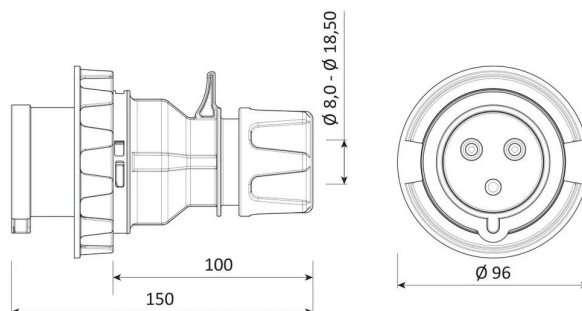
ГАБАРИТНЫЙ ЧЕРТЁЖ
