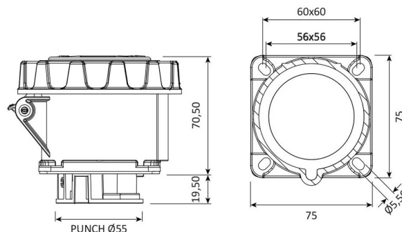
ГАБАРИТНЫЙ ЧЕРТЁЖ
