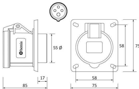
ГАБАРИТНЫЙ ЧЕРТЁЖ
