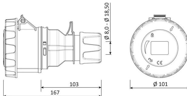
ГАБАРИТНЫЙ ЧЕРТЁЖ
